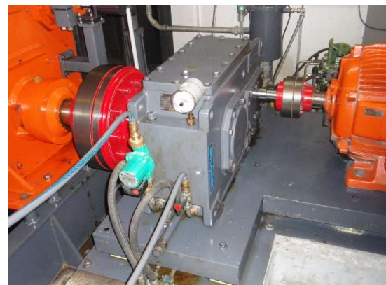
Getriebe dazwischen
